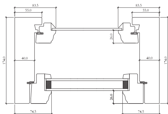
Vaakaleikkaus
