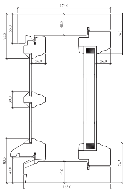
Pystyleikkaus
