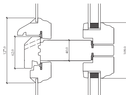
Pystyleikkaus
