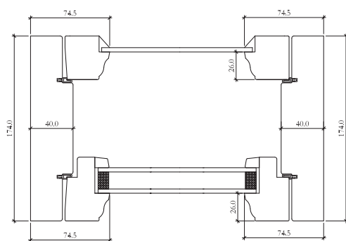
Vaakaleikkaus KARMIT
