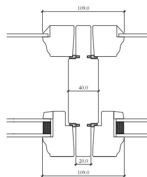
Vaakaleikkaus VÄLIKARMIT
