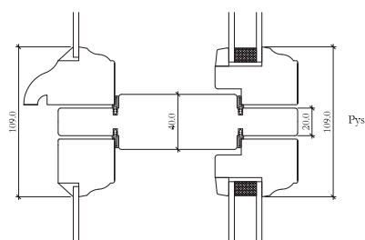
Pystyleikkaus
