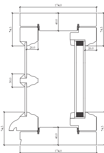
Pystyleikkaus
