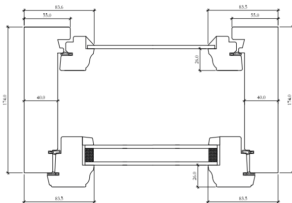
Vaakaleikkaus
