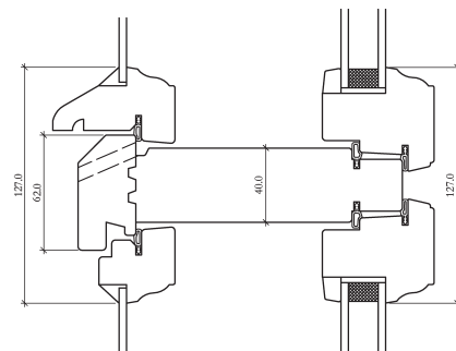
Pystyleikkaus
