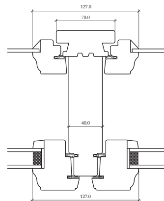
Vaakaleikkaus
