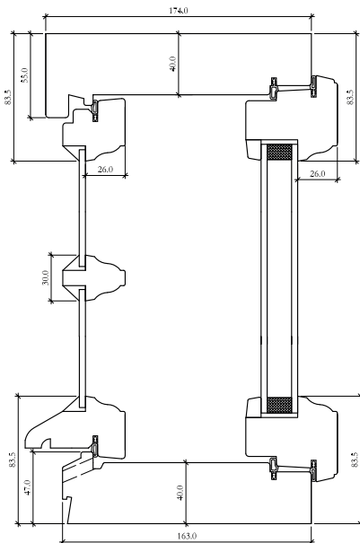
Pystyleikkaus
